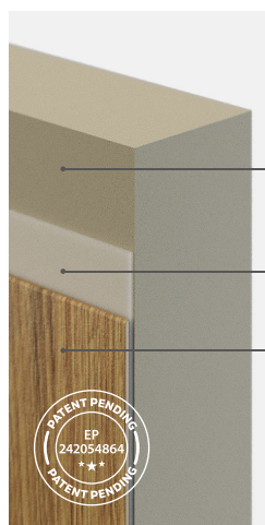
Průřez zárubní HYDRO PROTECT™
