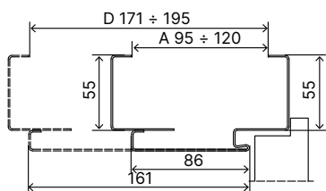
Rozsah zárubně
