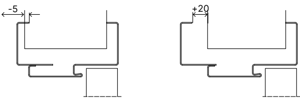
Rozsah regulace
