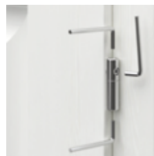
ajustarea balamalelor reglabile 3D
