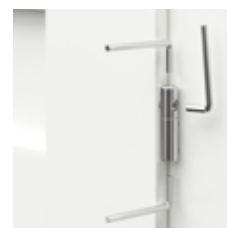
ajustarea balamalelor reglabile
