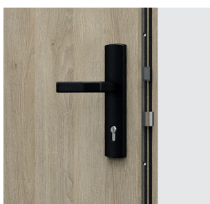
01 hákový zámok viacbodový systém Winkhaus
